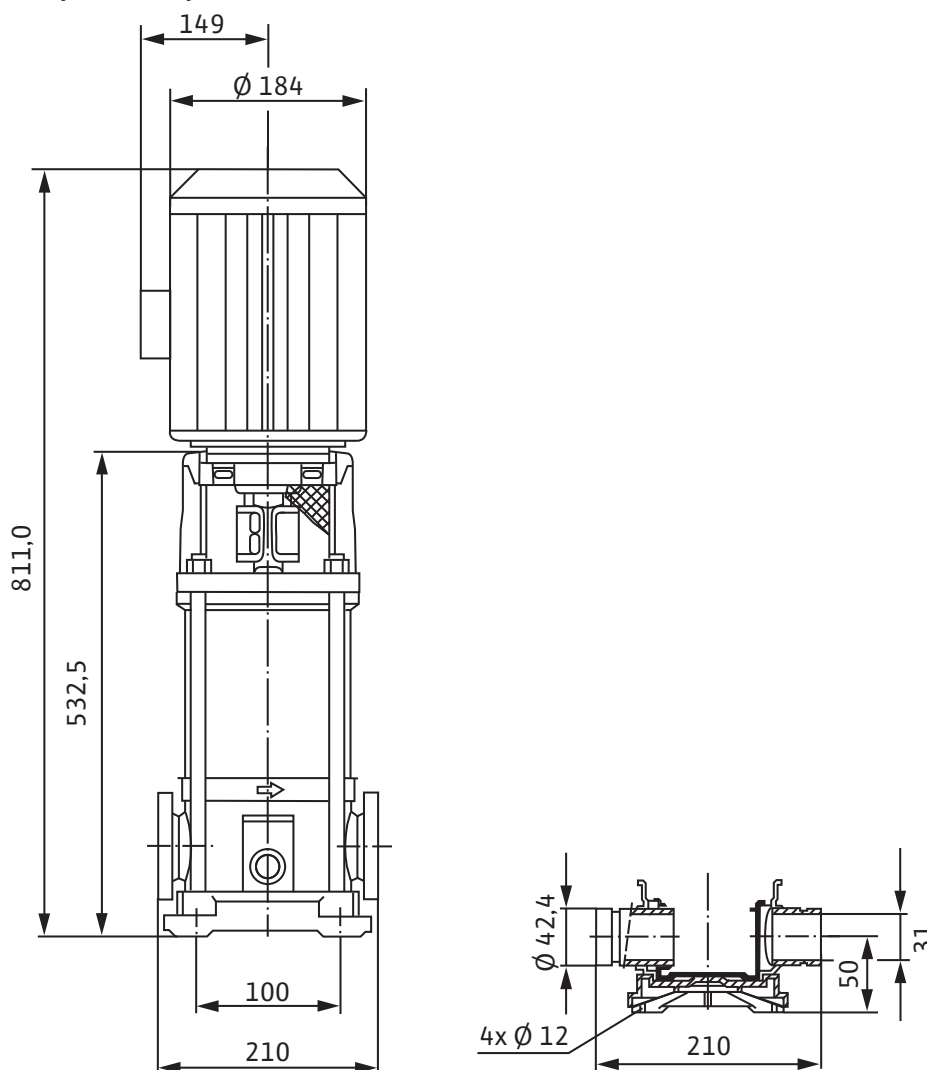
Габаритный чертеж
