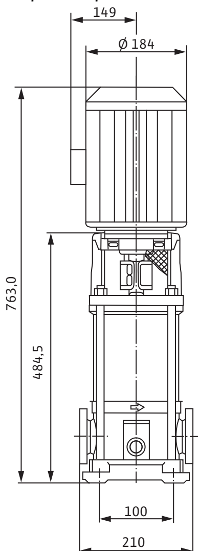
Габаритный чертеж
