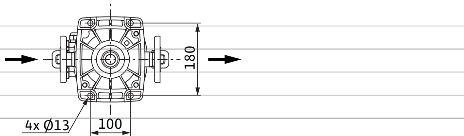
Габаритный чертеж
